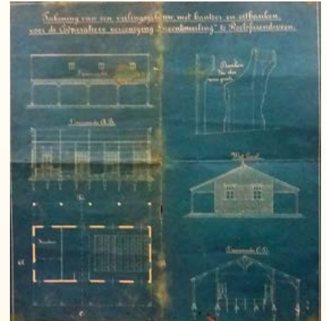
De bouwtekening van het veilinggebouw.
